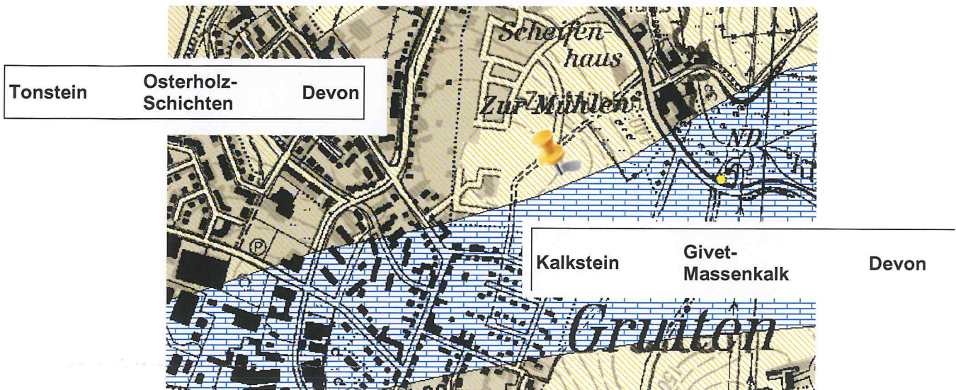
Abb. 1: Obere Grundwasserleiter im Untersuchungsraum
