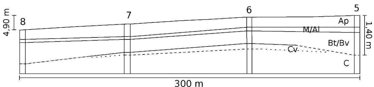
Abb. 6: Schematische Darstellung des Bodenaufbaus entlang des Sondageschnitts anhand der Geoprofile St. 5-8 (gespiegelt)
