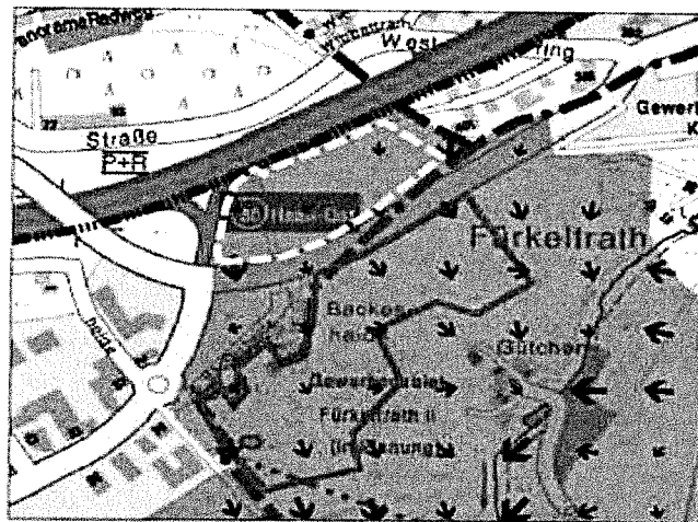
Abb. 5: Ausschnitt - Kaltluftdynamik im Untersuchungsgebiet Fückeltrath II (rotmarkiert) sowie nördlich der L 357 der Geltungsbereich des Bebauungsplans Nr. 193 (gelbmarkiert) (Quelle: Klimagutachten für das Ittertale in Solingen, S. 21, Abb. 8, Klimatologie – Geographisches Institut – Ruhr-Universität Bochum, 2015, erg. ISR 2018)
