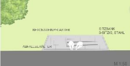
DETAIL SITZPLATZ
