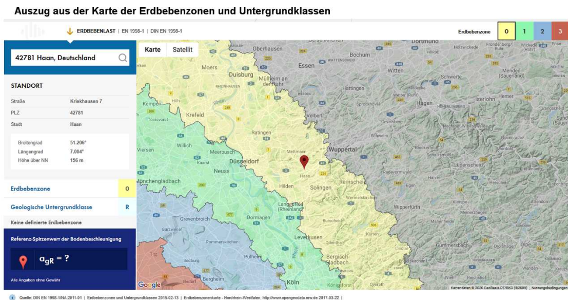
Abbildung 10: Auszug aus der Karte der Erdbebenzonen und Untergrundklassen
