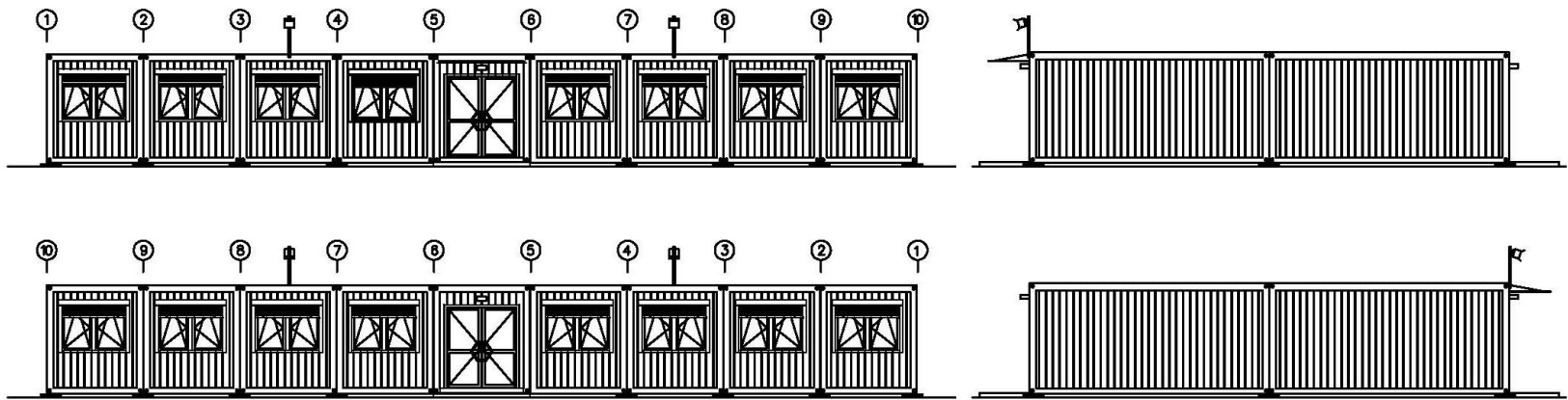
Interim 01 – Längsansichten und Queransichten
